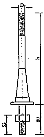
TIGE RENFORCEE (TR)
