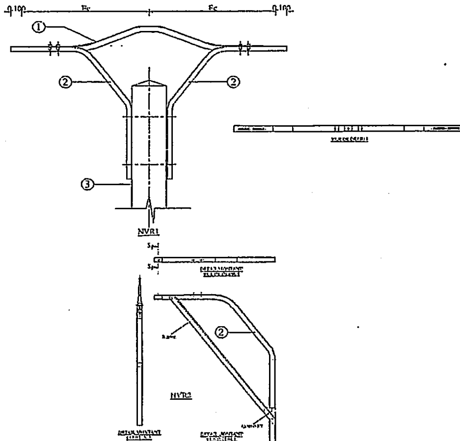
TYPES DE NAPPES VOUTE
