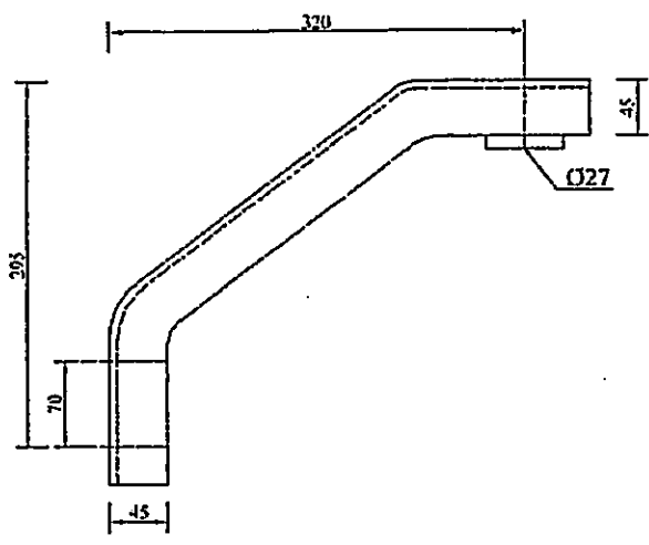
BRAS INCLINE RIGIDE (BIR)
