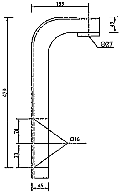
BRAS DE TETE RIGIDE (BTR)
